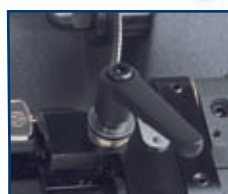
1 Sistema reversible de doble mordaza, a dos posiciones: a) duplicado de llaves de gorja. b) duplicado de llaves frontales.
